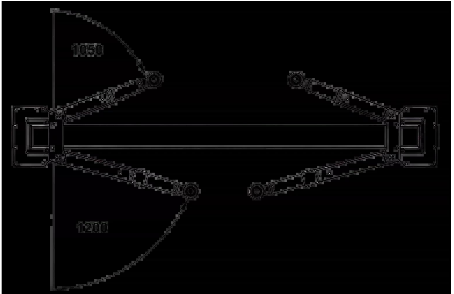
Ramiona robocze i zakres pracy Charakterystyka
