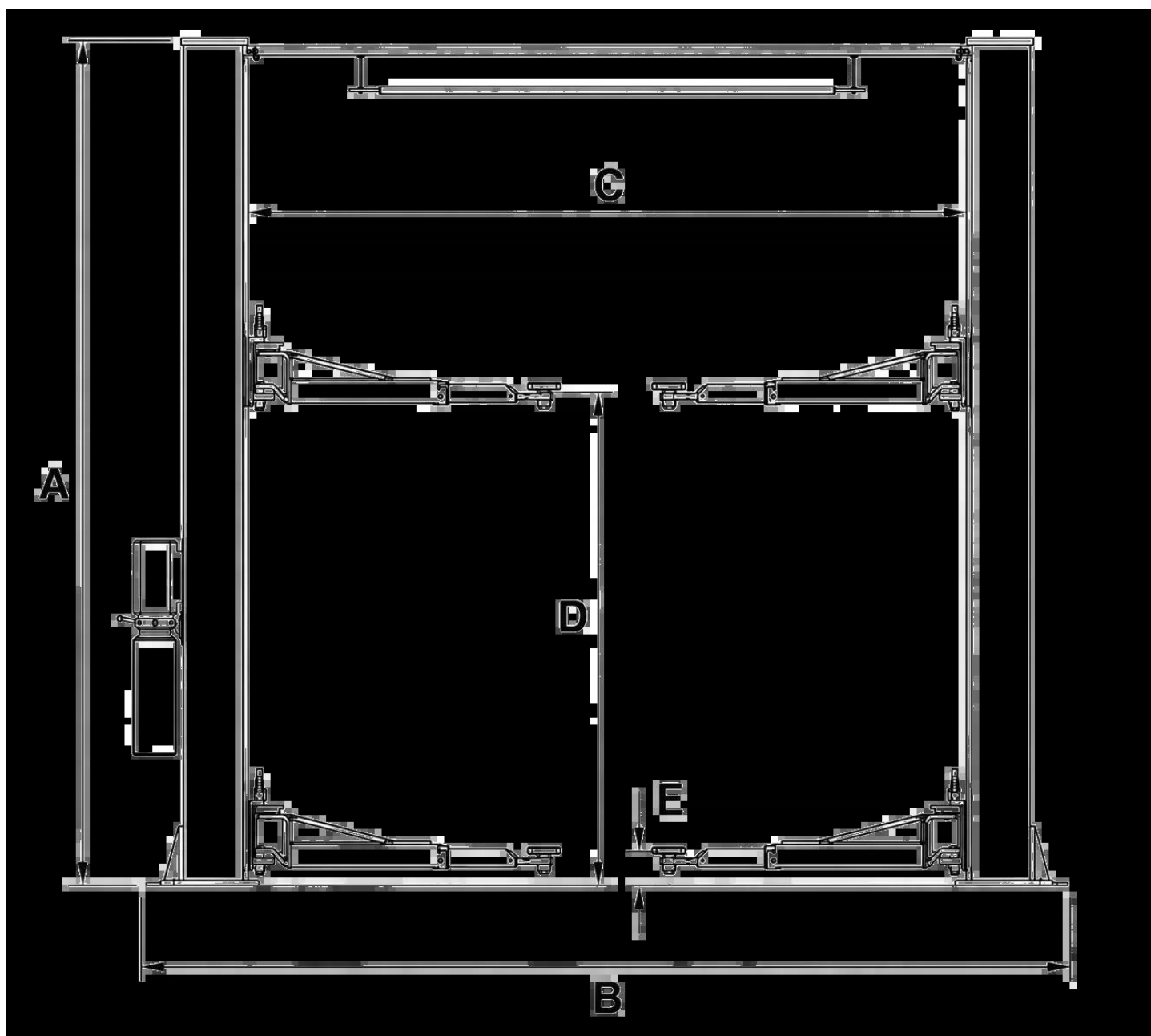
Schéma dimensionnel du pont élévateur avec traverse supérieure
