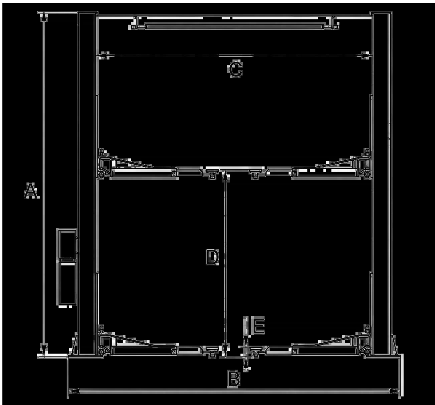
Schéma dimensionnel du pont élévateur avec traverse supérieure
